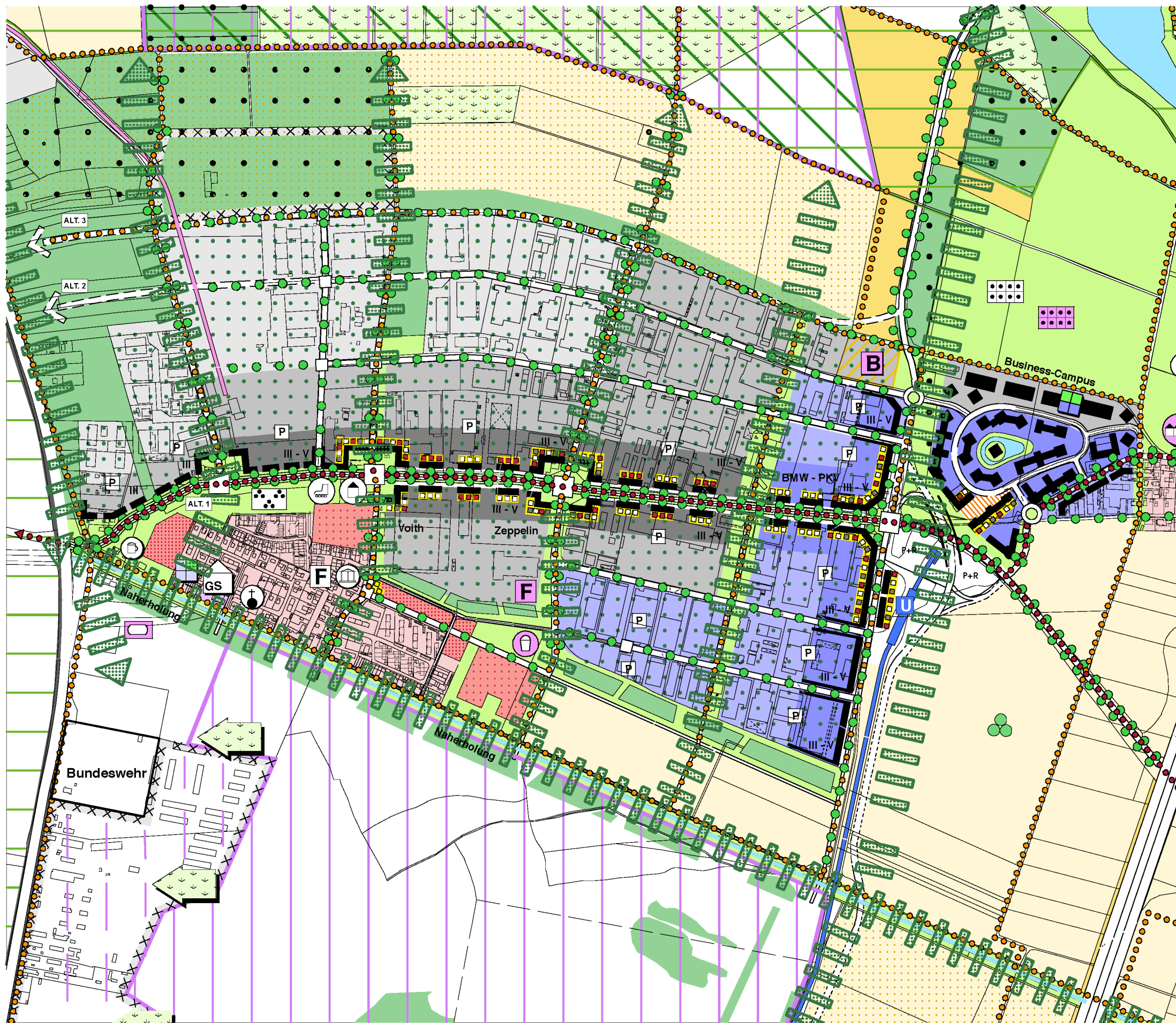
STADT GARCHING B. MÜNCHEN STADTENTWICKLUNGSPROZESS Gesamtentwicklungskonzept, Ausschnitt Hochbrück M 1:10.000
