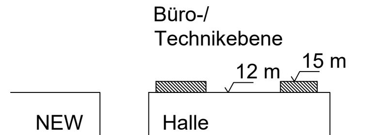
Systemschnitt A-A
